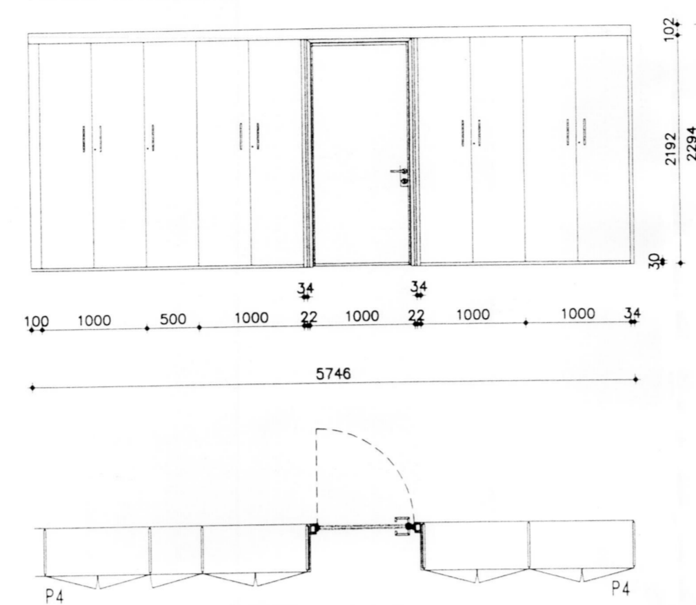
PROSPETTO TIPO P4 PARETE ATTREZZATA
