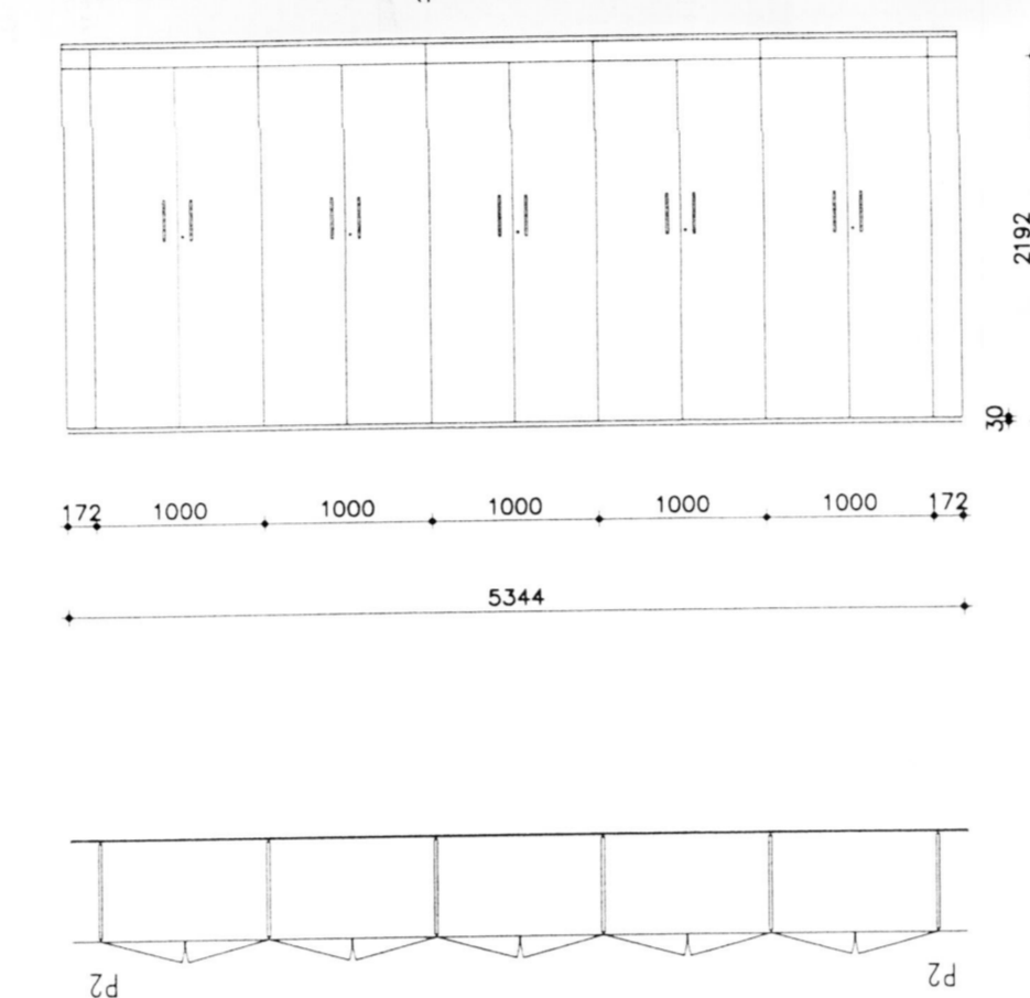
PROSPETTO TIPO P2 PARETE ATTREZZATA (prof. 600 mm.)
