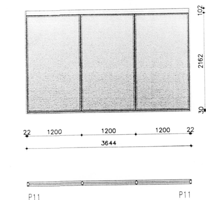
PROSPETTO P11 PARETE DIVISORIA ACIDATA
